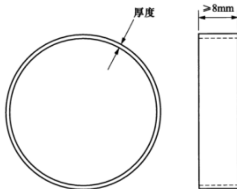
图 A.1 导管的环形试样
